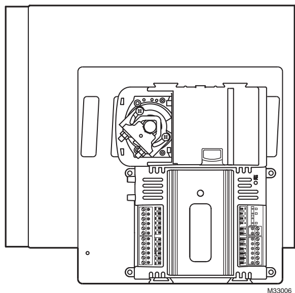
Fig. 11. D690 w Spyder Micro VAV
