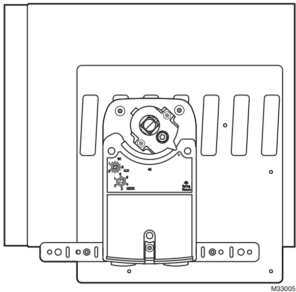
Fig. 10. D690 w MS7505.
